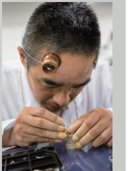
部品の反りや狂いを一つひとつ調整しながら組み立て。ミクロン単位の精度が要求されます。
